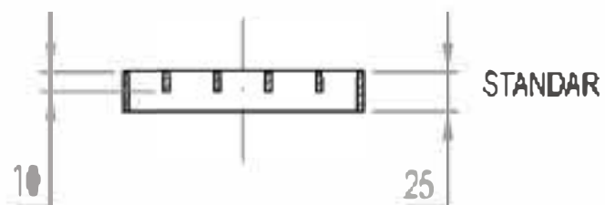
DETALLE PERFIL REJA ENTRAMADA MALLA 25X25 X2
